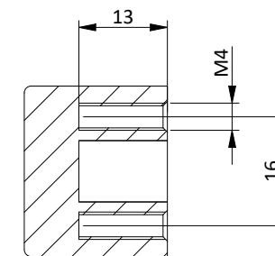
A-A ( 1 : 1 )
