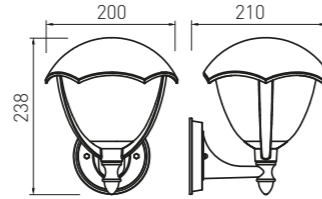
OS-GRA0UA-00
